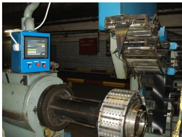
Установленные новый шкаф и панель управления (необходимость в огромном количестве кнопок отпала после модернизации интерфейса)
